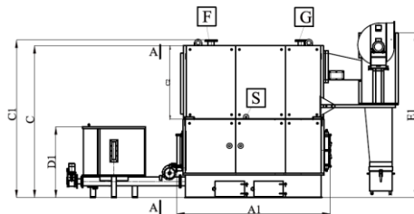
Seitenansicht
