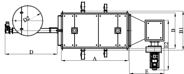
Vorderansicht
